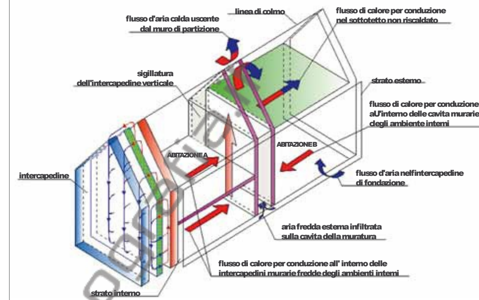
Fig. 9 Dinamica del thermal bypass in un muro di separazione tra ambienti riscaldati
