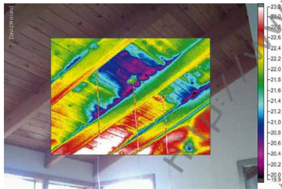
Esempi di thermal bypass in strutture a secco.
