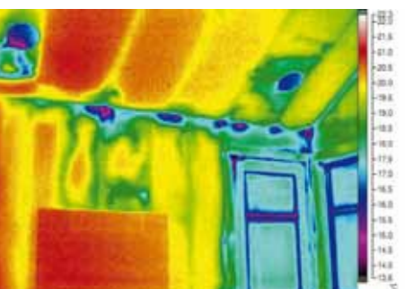
Esempi di thermal bypass in strutture a secco.
