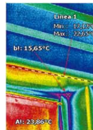
Immagine di un thermal bypass evidenziato in una struttura con intercapedine. Il flusso d'aria non entra all'interno dell'immobile, ma raffredda la muratura in corrispondenza del cassonetto dell'avvolgibile
